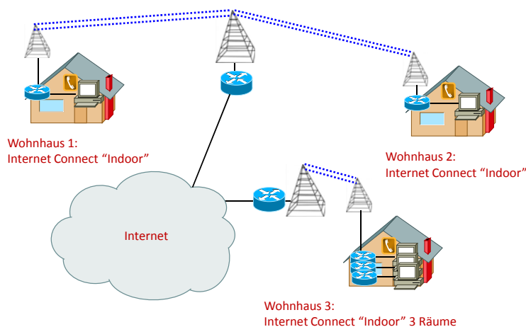
ENNSTAL [IT] „Internet Connect“ Privat/Indoor – schematische Darstellung
